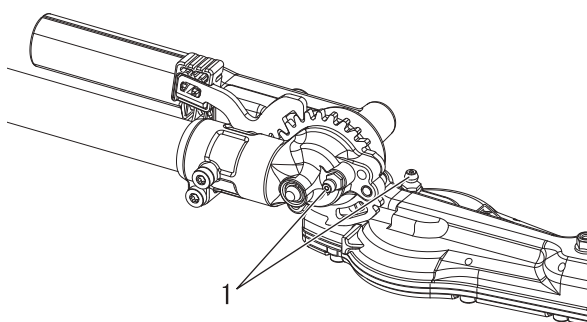
1. Raccordi di ingrassaggio della scatola degli ingranaggi
