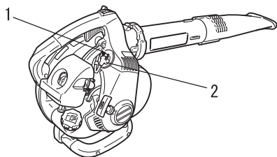
2. Zündkerzenstecker
