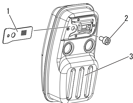
1. Funkenschutzsieb 3. Schalldämpfer
