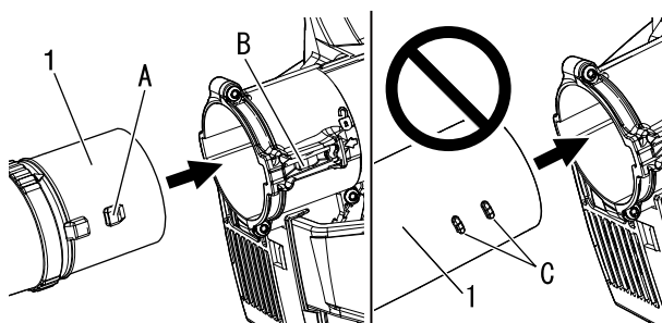
1. Blower pipe
